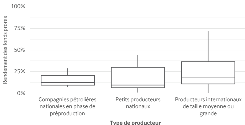
Figure 4 : Rendement des capitaux propres (ROE) par niveau de production et par région, 2015-19 154
