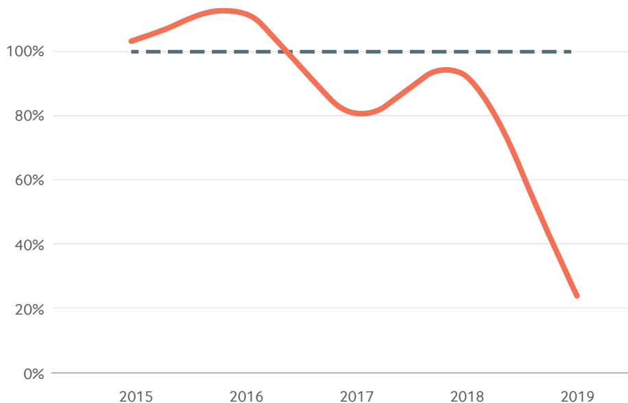
Figure 8 : Ratio de liquidité moyen par niveau de production et par région, 2015-2019 164
