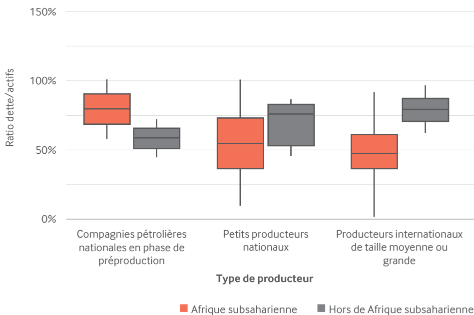
Figure 6 : Ratio moyen dette/actifs par niveau de production et par région, 2015-2019
